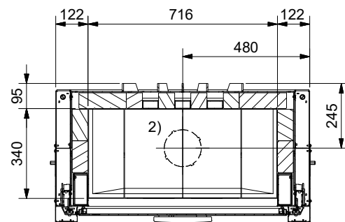
Grundriss Feuerstelle / Coupe sur foyer Sezione al piano fuoco / Layout fireplace
