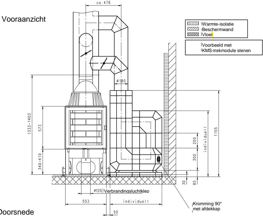
Doorsnede
