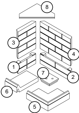
Tekening geldt voor hoekmodellen en 90° spitse hoekmodellen
