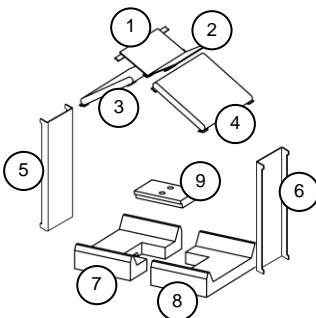
Tekening geldt voor tunnel toestellen
