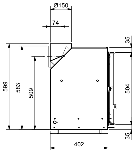
Seitenansicht / Vue de côté Vista laterale / Side view
