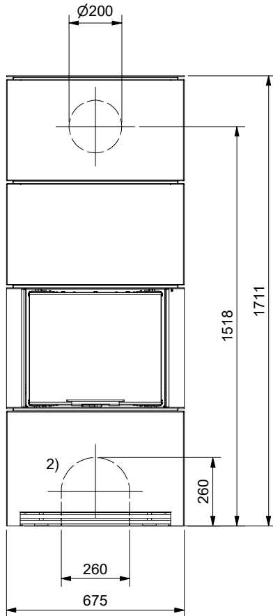
Frontansicht / Vue de face Vista frontale / Front view
